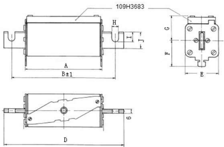
Dimensions(mm)安装尺寸示意图: (0EKN/155、1EKN/166、2EKN/170、3EKN/170)
